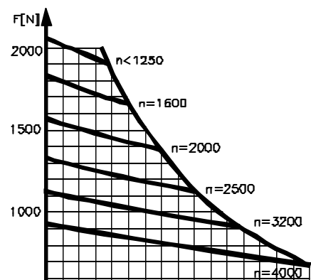
Silniki G 11.02-G11.05 – wyk. pionowe
