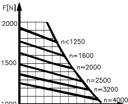
Silniki G 11.02-G11.05 – wykonania poziome
