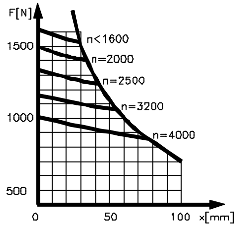
Silniki G 11.02-G11.05 – wyk. pionowe
