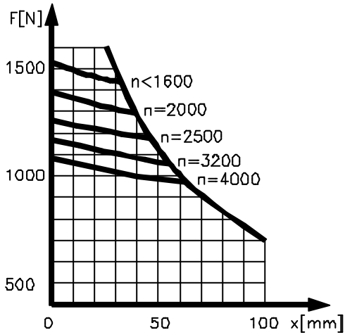
Silniki G 11.02-G11.05 – wykonania poziome
